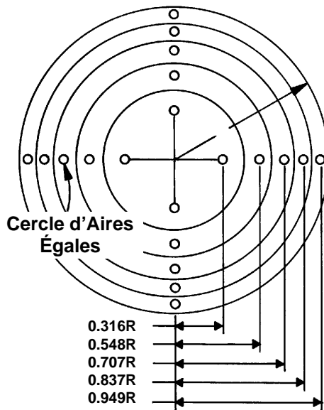
Points de traverses de conduits circulaires
