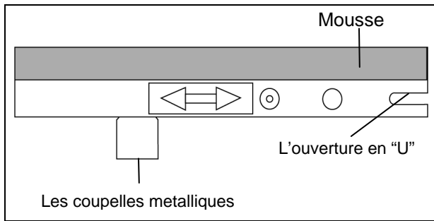
Figure 1 Canal du cadre de hotte
